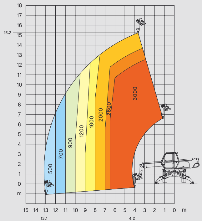
ROTACIÓN SOBRE ESTABILIZADORES CON CABRESTANTE 3 T
